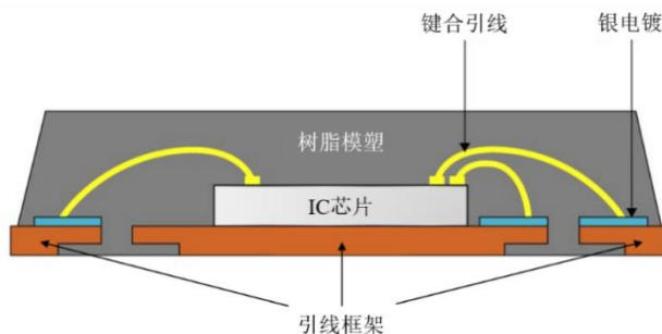
引线框架封装示意图
