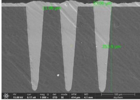
孔径50 μm，深度250 μm，AR~5
