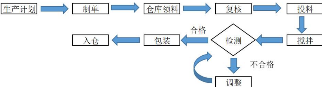
溶剂型产品工艺流程图
