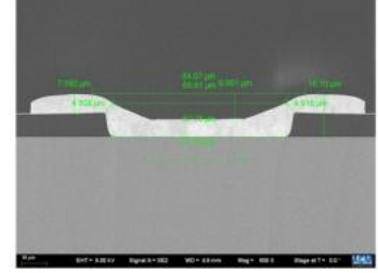
小孔形貌
