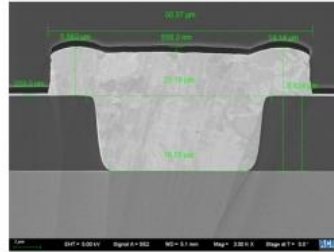
大孔形貌
