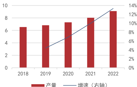
图表 5 近年来我国覆铜板产量情况（单位：亿平方米）
