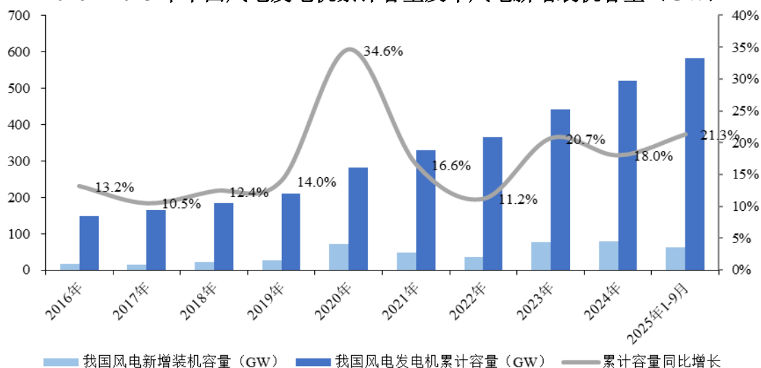
2016—2025 年中国风电发电机累计容量及年风电新增装机容量（GW）
