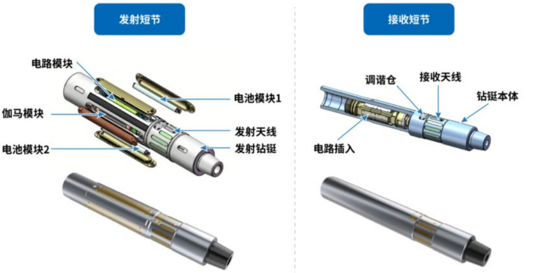
近钻头随钻测量系统结构示意图（包括发射短节、接收短节两部分）
