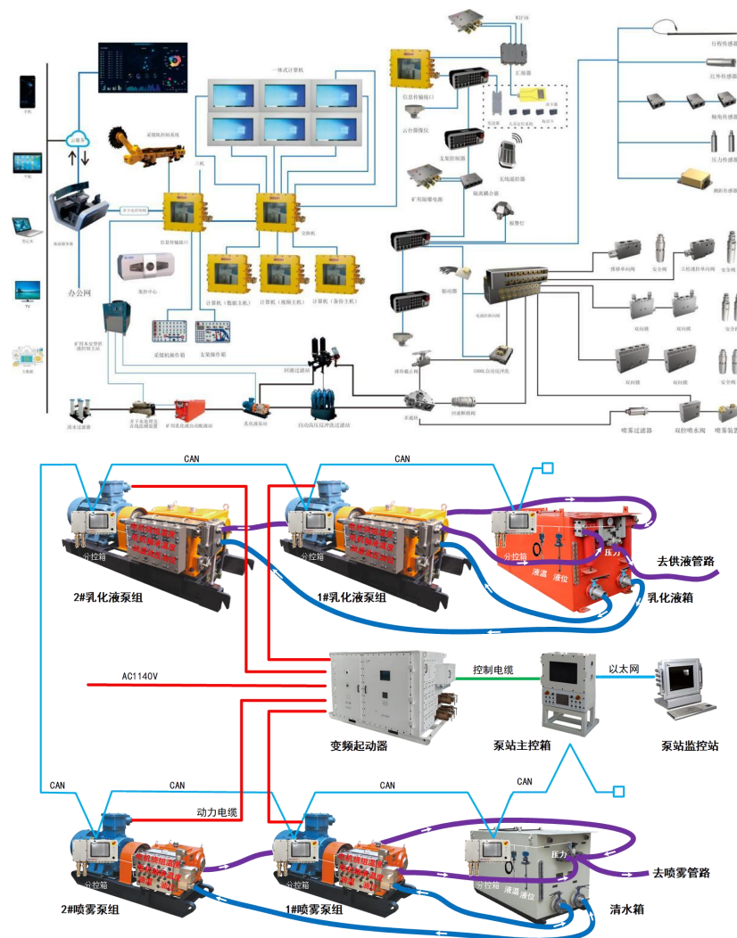
发行人的智能综采系统部分子系统示意图
