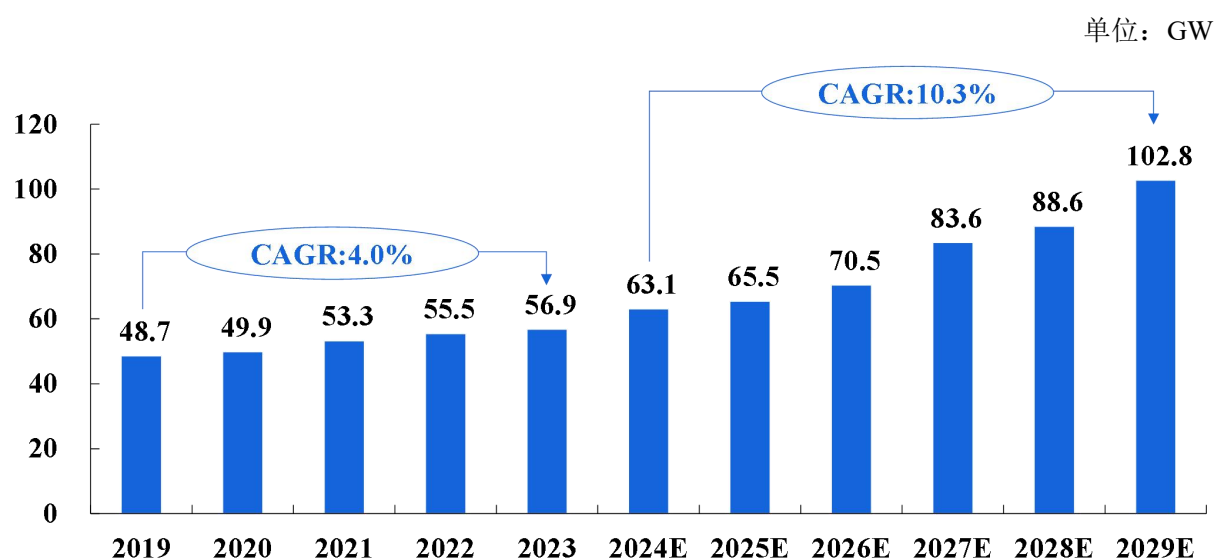
中国核能发电在运装机容量
