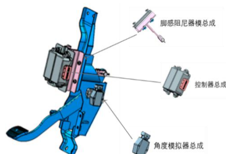
具有能量回收功能的电子踏板总成
